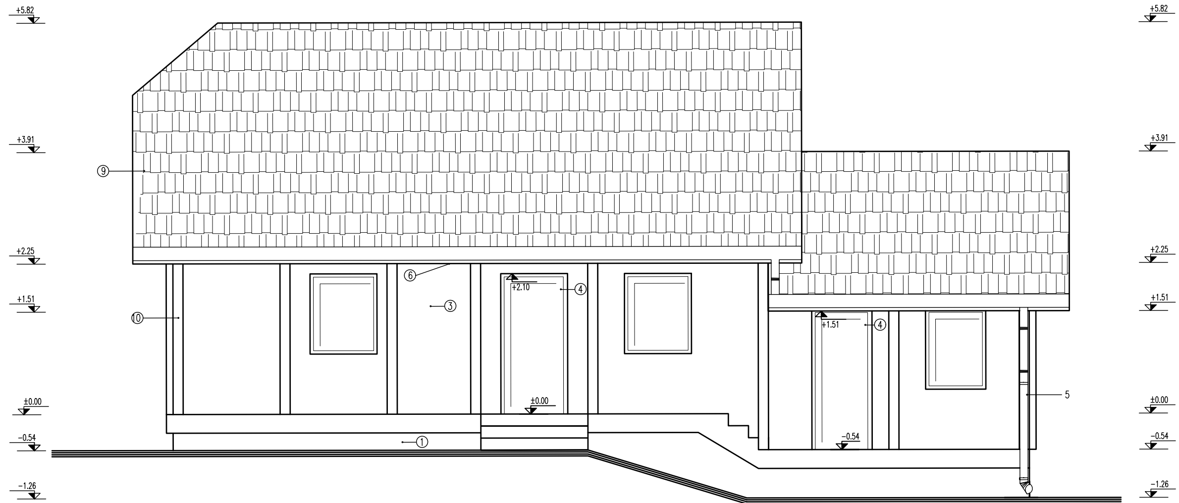
FATADA SUD EST FATADA LATERAL DREAPTA SCARA 1:50
